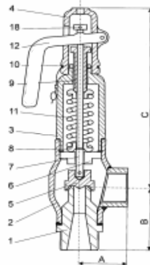
AVEC LEVIER
